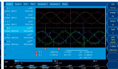
在两个波形页面中的 8 个信号的采样值显示
